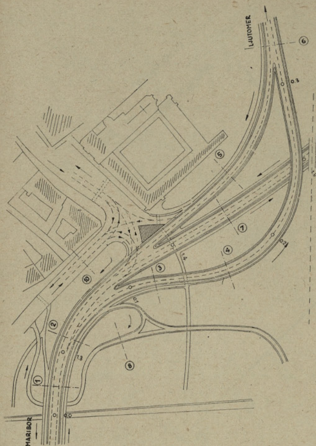
Sl. 4. Detajl situacije na levem bregu
