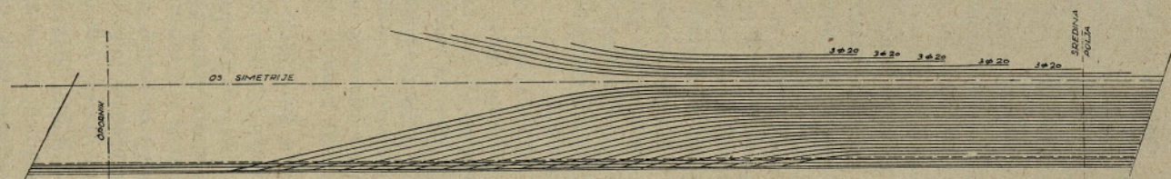
Sl. 19. Prečni prerez in razpored armature v spodnji plošči
