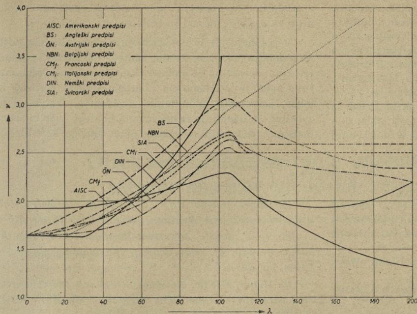
Slika 7. Diagram \nu - \lambda po različnih predpisih za Je 37 ( \sigma_{pl} = 2,3 \text{ t/cm}^2 ).
