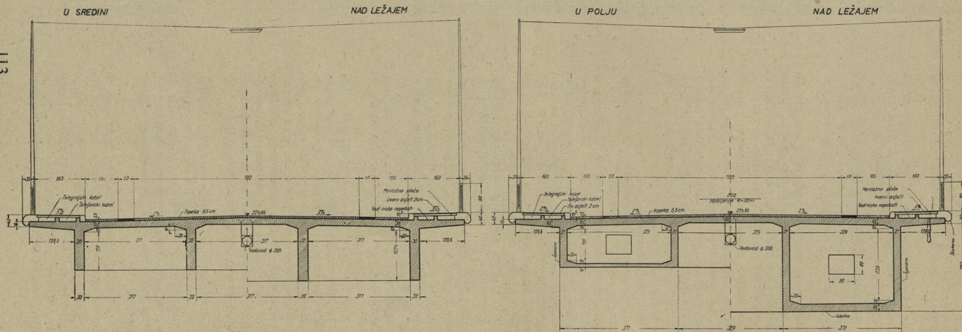
Sl. 7. Prečna prereza
