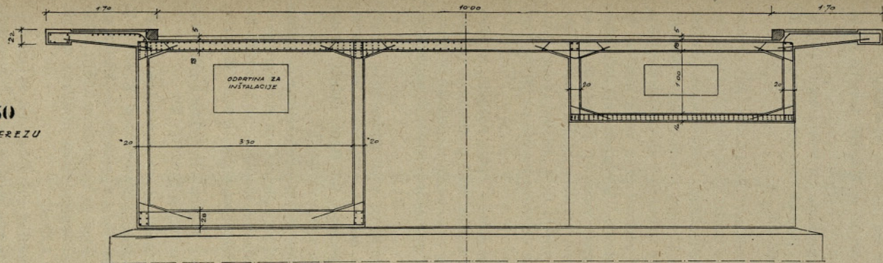
RAZPOREDITEV POZIT ARMATURE V SPODNJI PLOŠČI
