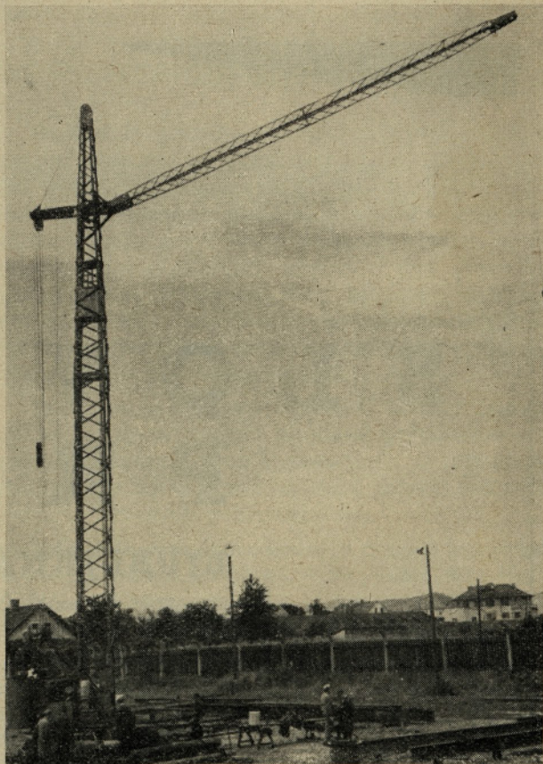
Varjeni stolpni žerjav »Krpan«, proizvodnja podjetja SKIP, Vižmarje pri Ljubljani, teža 8,9 t, obtežba 3,5 t, nosilnost 1350 kg, skupna moč elektromotorjev 13,3 kW, najvišji položaj kavlja 22,5 m, hitrost dviganja 44,9 m/min., pomol od 6,2 do 12,2 m. Prevoz žerjava z gradbišča na gradbišče je omogočen s tovornim avtomobilom tako, da je vodoravno položen stolp pritrjen na kamion, pod voziček žerjava pa je vložena posebna os z gumijastimi kolesi. Dvi-ganje stolpa v vertikalni legi se izvrši brez uporabe ka-kršnihkoli pomožnih naprav s pomočjo električnega vitla, ki je montiran na žerjavu
