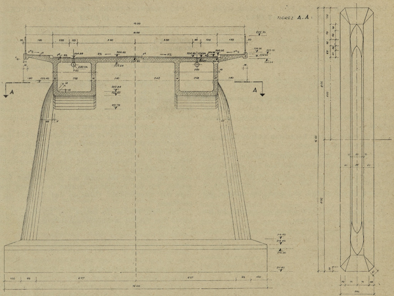
Sl. 22. Prečni prerez med vmesnimi podporami in tloris rečnega stebra
