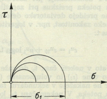
Slika 5. Enoosni kompresijski preizkus
