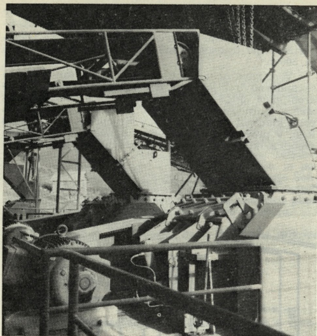
Sl. 4. Primarno in sekundarno drobljenje materiala
