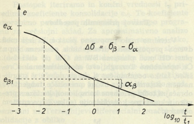
Slika 1. Konsolidacijska krivulja pri edometričnem preizkusu
