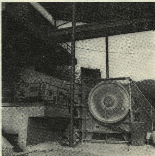
Sl. 3. Izločevalna vibracijska rešetka in predhodni čeljustni drobilnik
