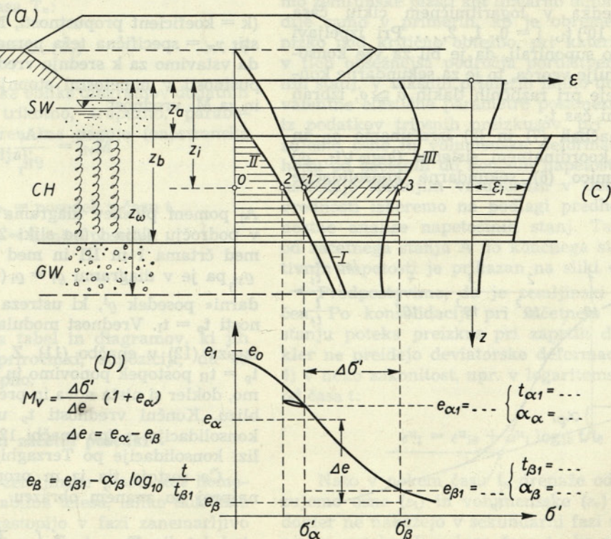
Slika 2. (a) diagrami navpičnih tlakov \sigma_2 = \sigma ; (b) krivulja stisljivosti edometričnega preizkusa; (c) diagram specifičnih deformacij
