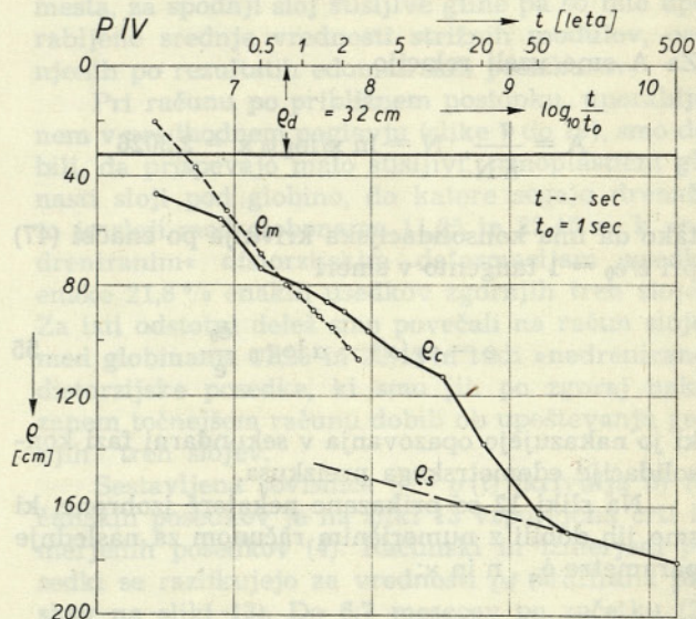
Slika 10. Izmerjeni (črtkana linija) in aproksimativno izračunani tok posedkov za točko 4 (slika 6). Reproduciranje po Gaberčevi in Vidicu (1977) s podaljšanjem črte izmerjenih posedkov po meritvah v letu 1977
