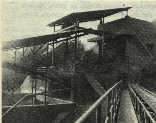
Sl. 2. Pogled na predhodno drobilnico in vmesno deponijo materiala
