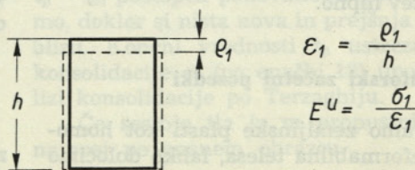
Slika 5. Enoosni kompresijski preizkus
