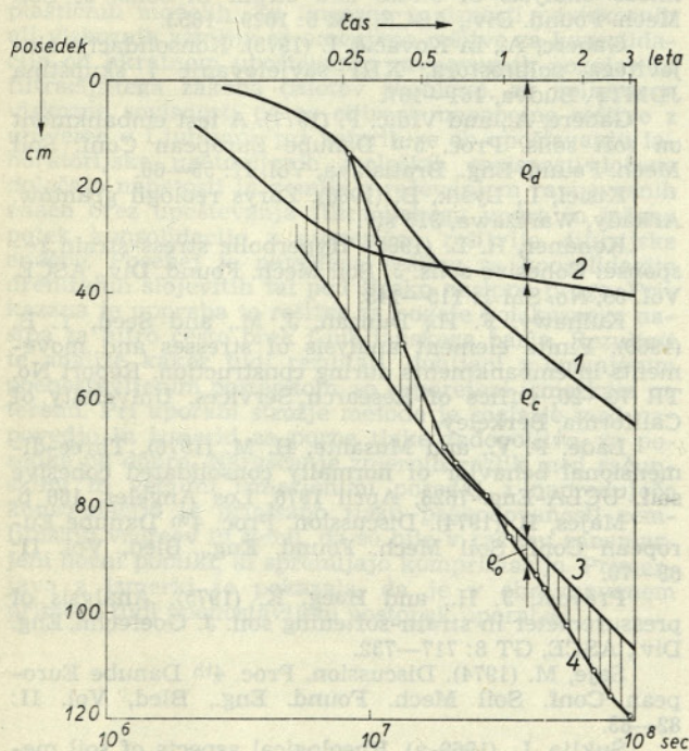
Slika 13. Primerjava izračunanih in izmerjenih posedkov za točko 1 (slika 6): (1) konsolidacijski posedki \varrho_c , (2) čisti »nedrenirani« distorzijski posedki \varrho_d , (3) = (2) + (1), (4) izmerjeni posedki, (5) = (4) - (3)
