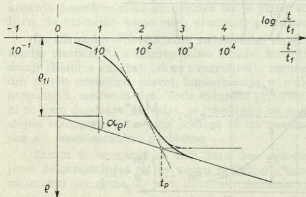
Slika 3. Črta sekundarnih posedkov \varrho_i = \varrho_{1i} + \alpha_{\varrho i} \cdot \log_{10} t/t_1 in priključek črte primarne konsolidacije nanjo
