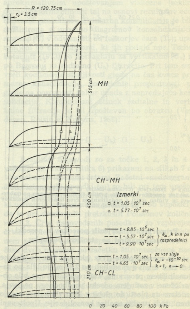
Slika 12. Izračunane izohrone vzdolž dreniranih slojev
