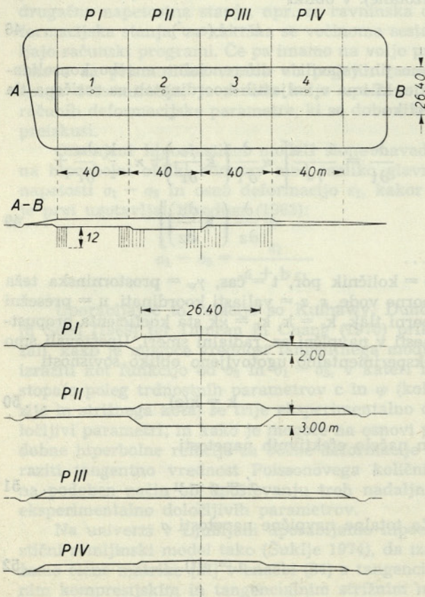
Slika 6. Tloris in profili polizkusnega nasipa na Ljubljanskem barju
