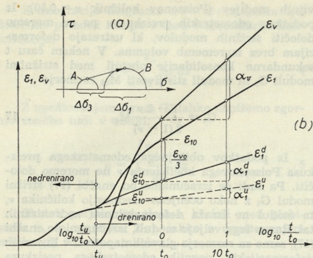
Slika 4. Konsolidacijske krivulje pri triosnem preizkusu
