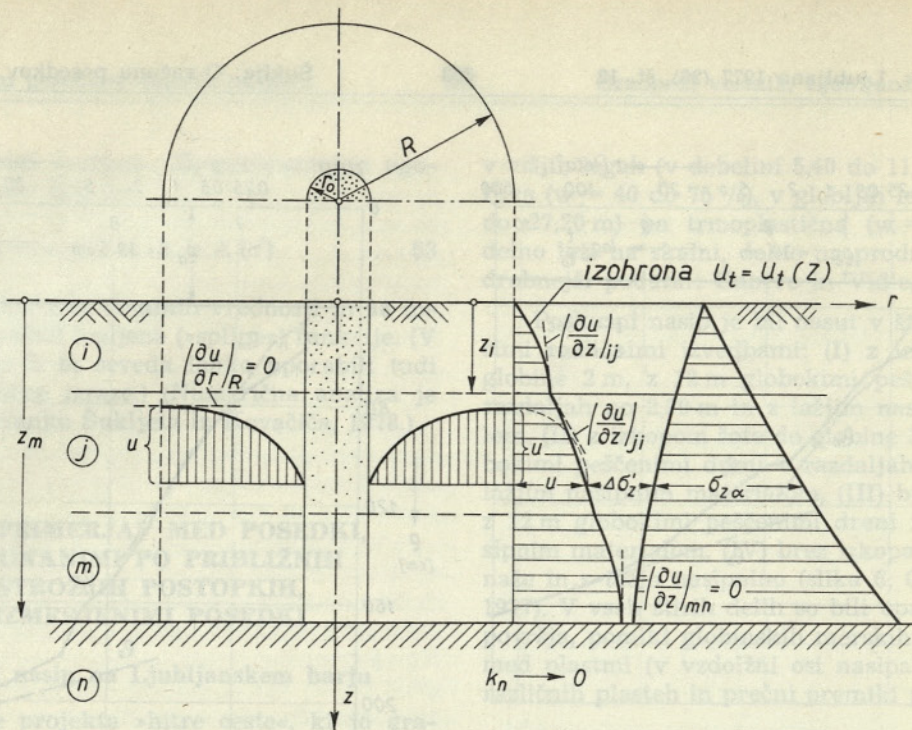
Slika 11. Robni pogoji za numerični račun konsolidacije dreniranih slojev
