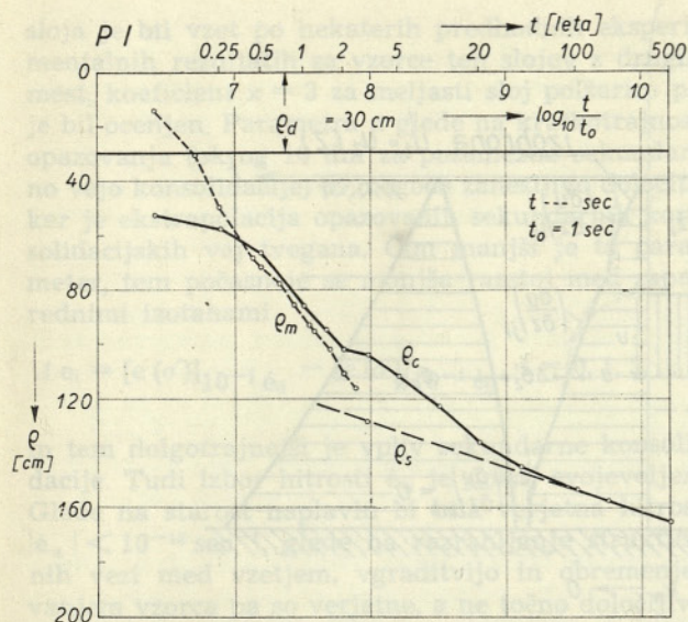
Slika 7. Izmerjeni (črtkana linija) in aproksimativno izračunani tok posedkov za točko 1 (slika 6). Reproduciranje po Gaberčevi in Vidicu (1977) s podaljšanjem črte izmerjenih posedkov po opazovanjih v letu 1977
