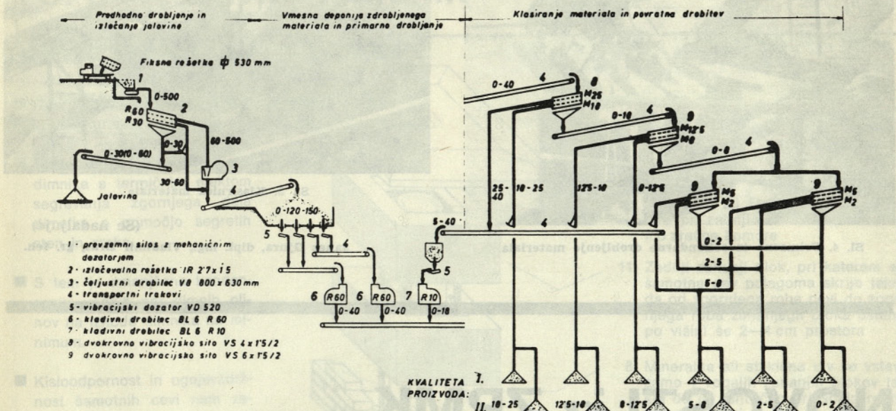
Sl. 1. Tehnološka shema separacije
