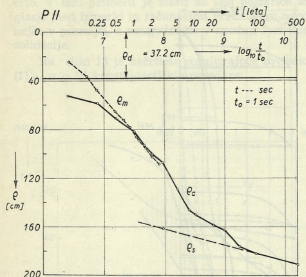
Slika 8. Izmerjeni (črtkana linija) in aproksimativno izračunani tok posedkov za točko 2 (slika 6). Reproduciranje po Gaberčevi in Vidicu (1977) s podaljšanjem črte izmerjenih posedkov po opazovanjih v letu 1977
