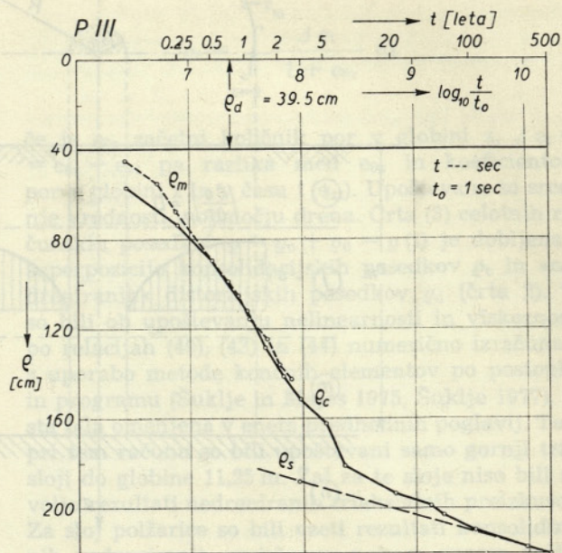
Slika 9. Izmerjeni (črtkana linija) in aproksimativno izračunani tok posedkov za točko 3 (slika 6). Reproduciranje po Gaberčevi in Vidicu (1977) s podaljšanjem črte izmerjenih posedkov po opazovanjih v letu 1977
