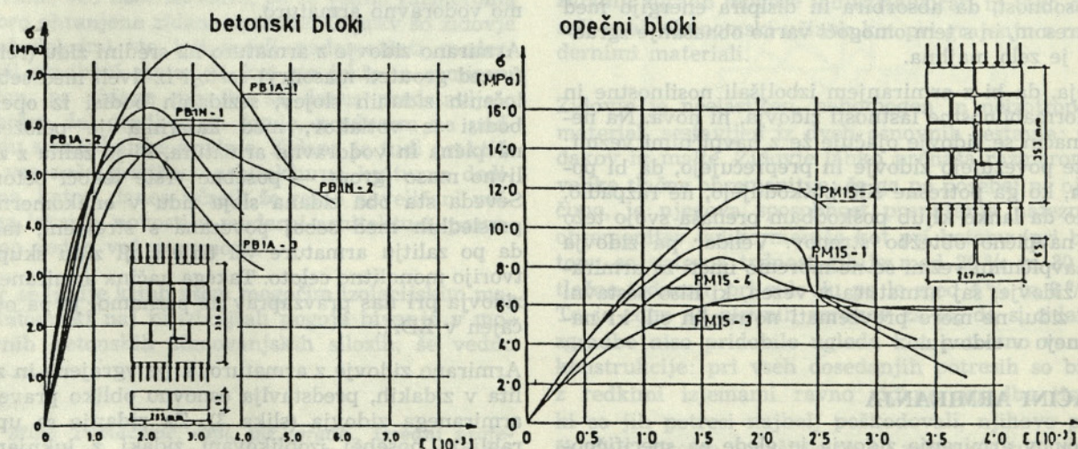
Slika 4. Delovni diagrami zidovja pri tlačnih obremenitvah (Tomažević in Žarnić, 1984, 1985)
