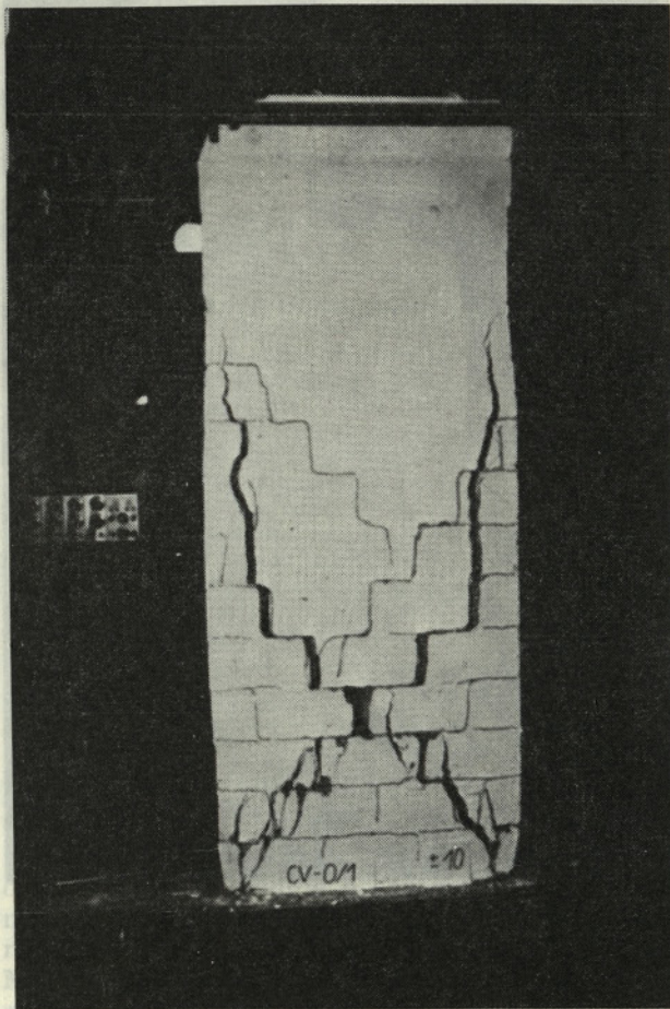
Slika 14. Strizna porušitev upogibno armiranega zidu brez strizne armature
