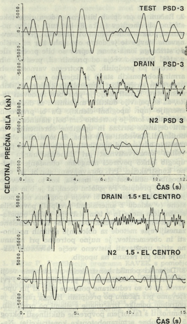
Slika 5. Časovni odziv celotnih prečnih sil spodaj
