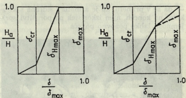
Slika 7: Mehanizem delovanja strižne armature (Tomažević, 1987)
