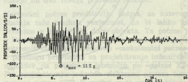
Slika 5. Sintetični akcelerogram
