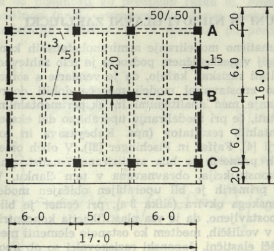
Slika 1. Tloris in prerez stavbe
