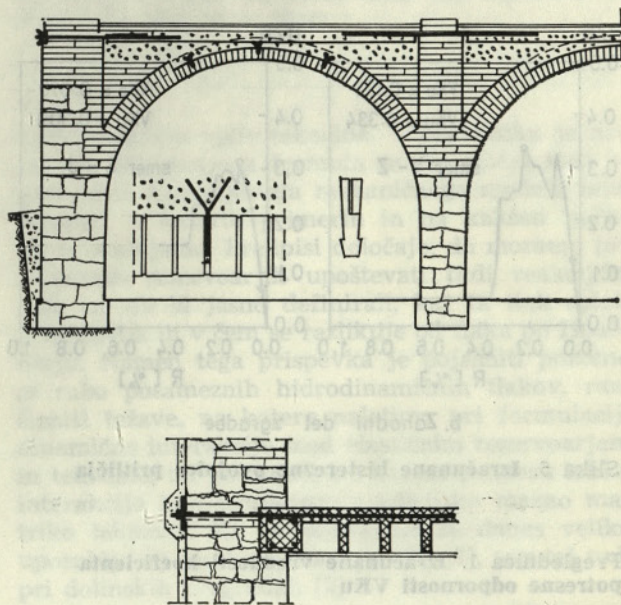
Slika 4. Skica ojačitve opečnega oboka in detajla sidranja novih plošč v zidove
