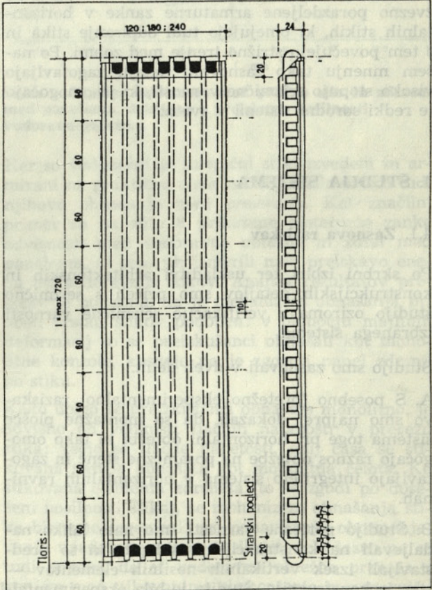
Slika 4. Stropni element
