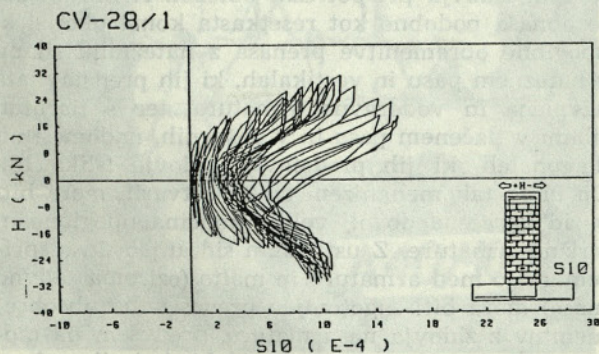
Slika 11. Histerezne zanke odvisnosti med vodoravno silo in specifičnimi deformacijami navpične armature (Tomažević in sod., 1986)
