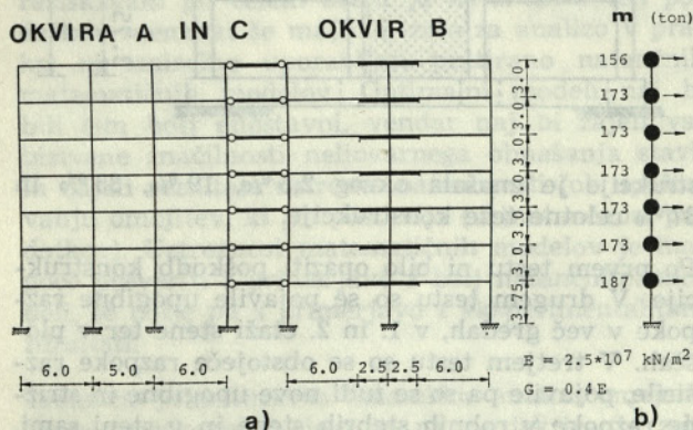
Slika 3. Matematični model konstrukcije:
