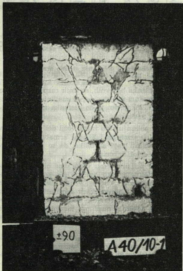
Slika 8. Razporeditev razpok pri strižni poružitvi vodoravno armiranega zidu
