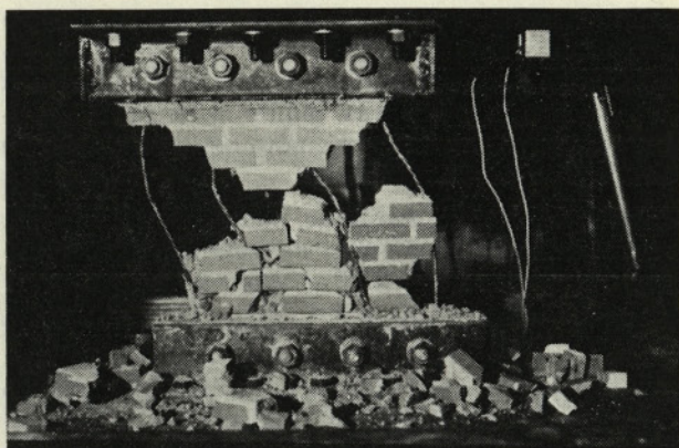
Slika 6: Strižna porušitev zidu, armiranega z navpično armaturo
