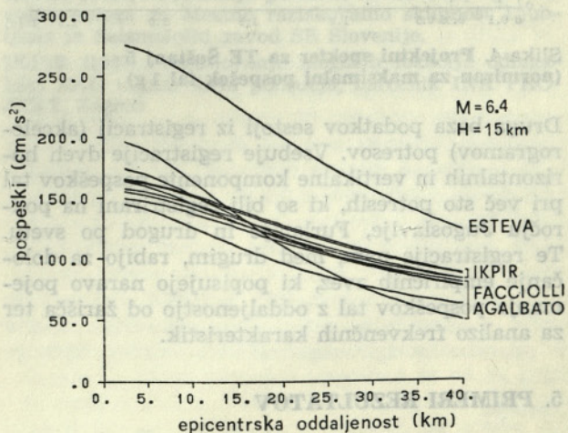
Slika 3. Primerjava atenuacijskih zvez za M = 6.4 in H = 15 km
