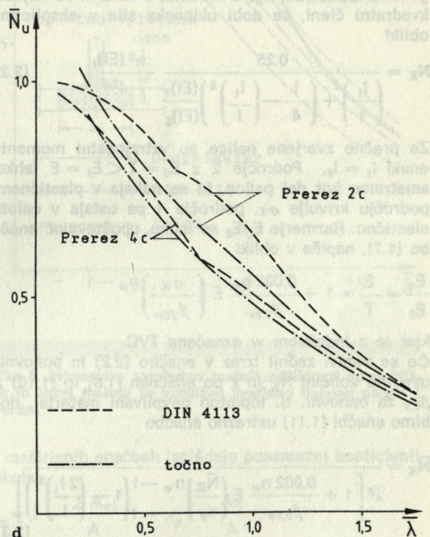
Slika 5. Primerjava mejne nosilnosti nezvarjenih tlačnih palic, določene po Dangelmaierjevi metodi in DIN 4113 s točnimi vrednostmi
