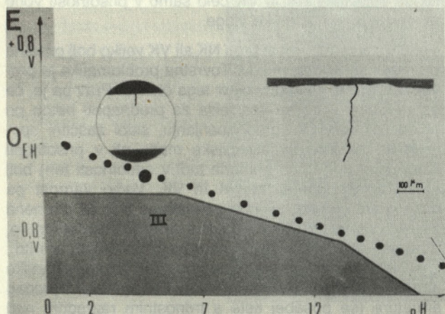
Slika 6. Vodikova krhkost v polju III, kjer je jeklo imuno pred korozijo (katodno zaščiteno). Vodikova krhkost pa se lahko pojavi tudi v polju I in IV (označeno z manjšimi pikami)
