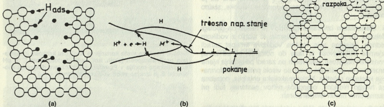
Slika 3. Vzemno delovanje napetostne korozije in vodika v napetostni razpoki
