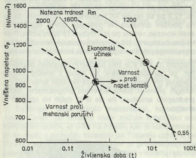
Slika 9. Življenjska doba patentirane žice v korozijskem mediju, ki povzroča NK, v odvisnosti od vnesene napetosti
