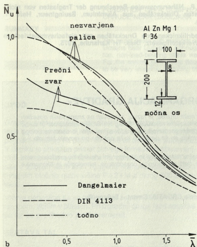
Slika 7. Primerjava rezultatov mejnih nosilnosti po približnih in točni metodi za tlačeno palico s prečnim zvarom v sredini
