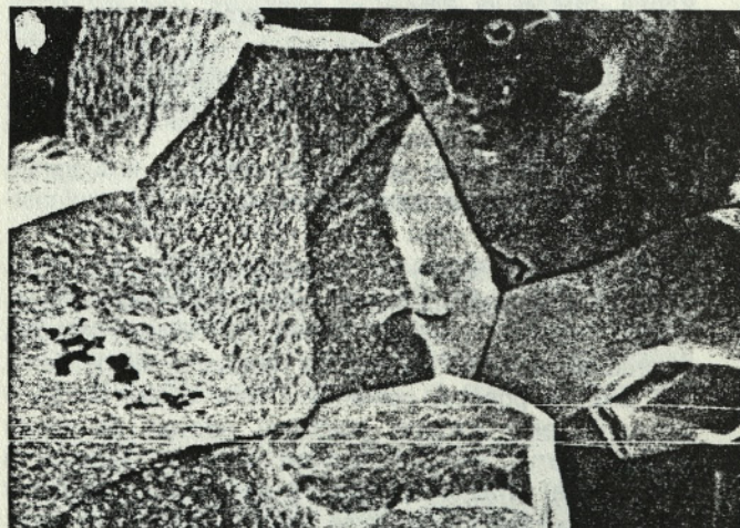
Slika 2. Interkristalno napetostno pokanje zaradi številnih depozitov po kristalnih mejah zrn
