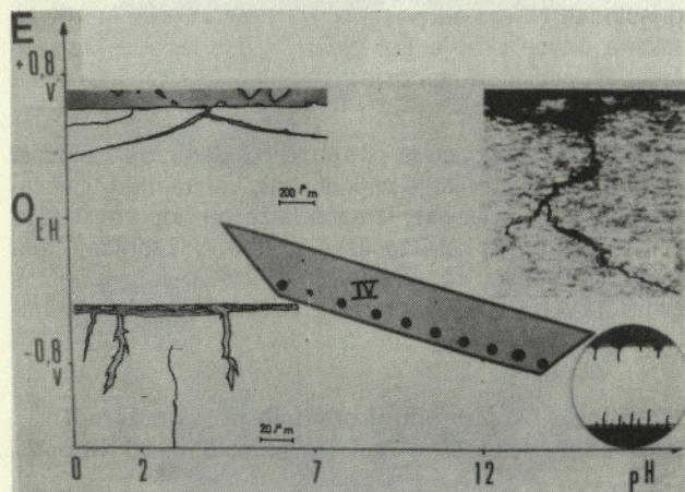
Slika 7. Napetostno korozijsko pokanje prednapete armature v področju IV, katero pa je lahko podprto še z vodikovo krhkostjo
