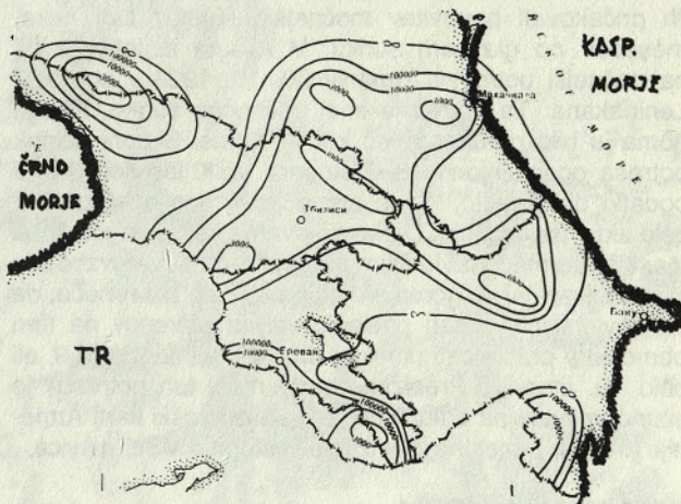
Slika 4. Prognoistična seizmološka karta za potrese 9. stopnje MSK
