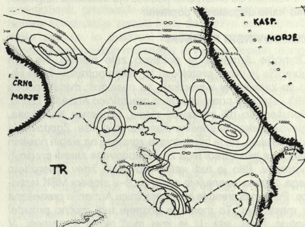
Slika 3. Prognoistična seizmološka karta za potrese 8. stopnje MSK
