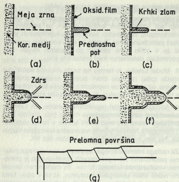
Slika 1. Mehанизem nastajanja interkristalne napetostno korozijske razpoke
