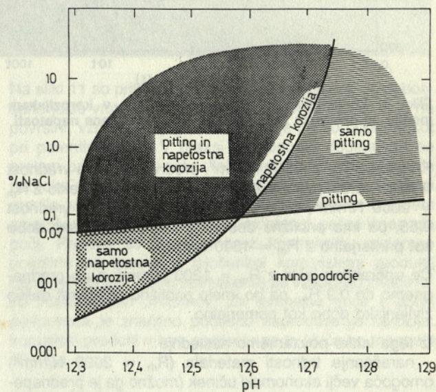
Slika 8. Vpliv pH betona in deleža kloridov na nastajanje pittinga ter napetostne korozije
