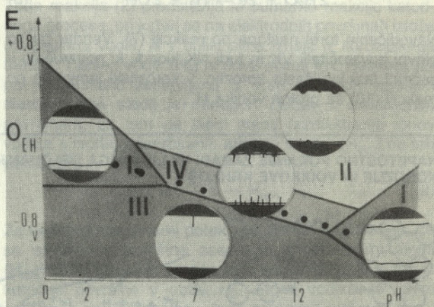
Slika 4. Različne vrste korozije in vodikova krhkost, ki nastajajo na prednapetih jeklih, kot funkcija potenciala E in pH korozijskega medija v Pourbaix ravnotežnem diagramu (potencial E je izražen proti vodikovi elektrodi – E_H )
