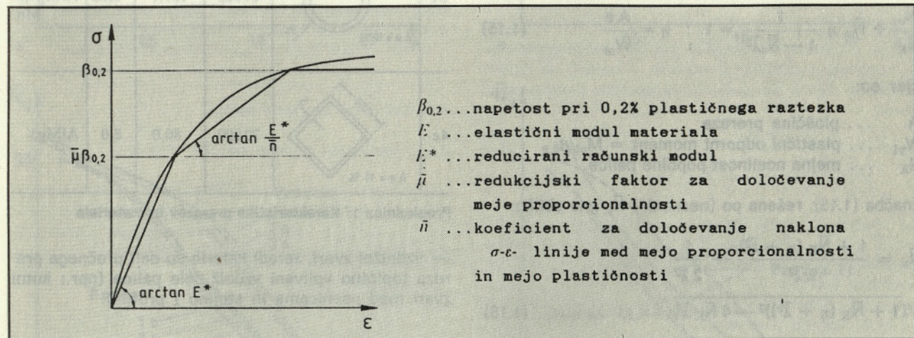
Slika 3. Tridelni sekantni opis \sigma - \varepsilon diagrama aluminijastih legur
