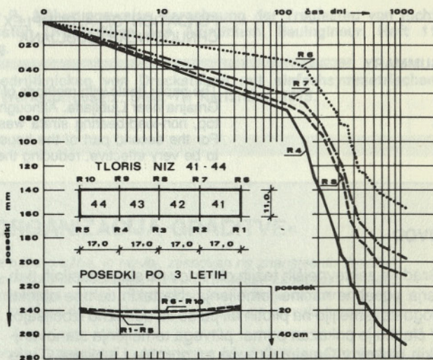
Slika 2. Krivulja posedkov
