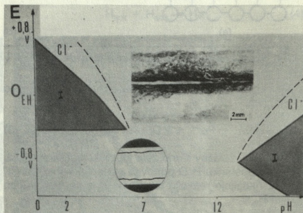
Slika 5. Splošna korozijska jekla v polju I
