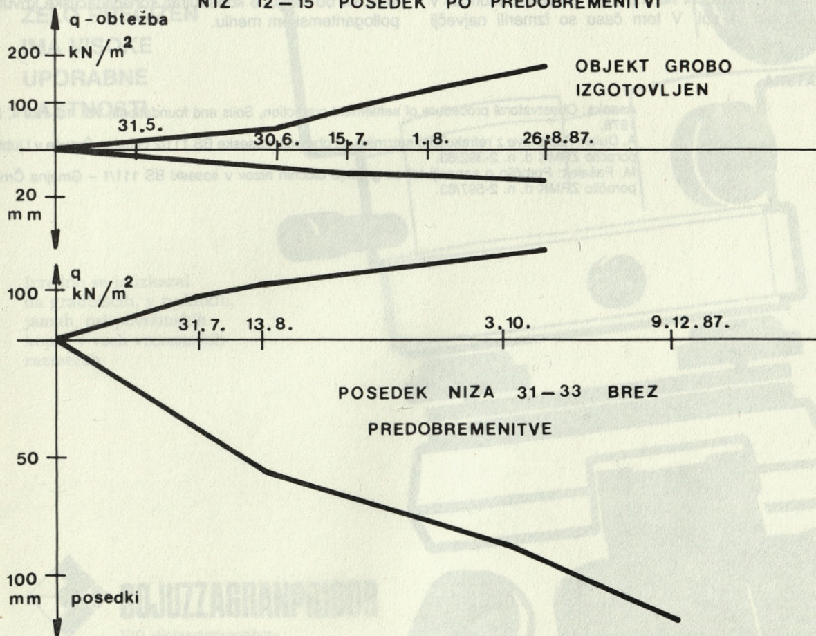
Slika 3. Primerjava posedkov: preobremenitev, brez preobremenitve
