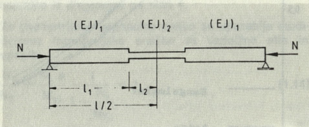
Slika 6. Sistem tlačene palice s prečnim zvarom v sredini
