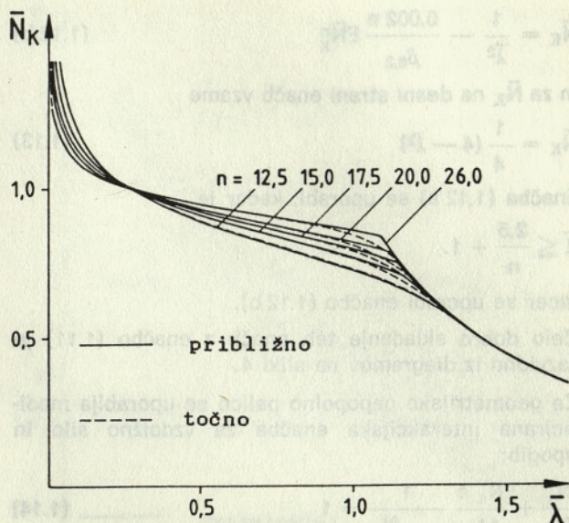
Slika 4. Primerjava točnega in približnega poteka krivulj \bar{N}_K - \bar{\lambda}
