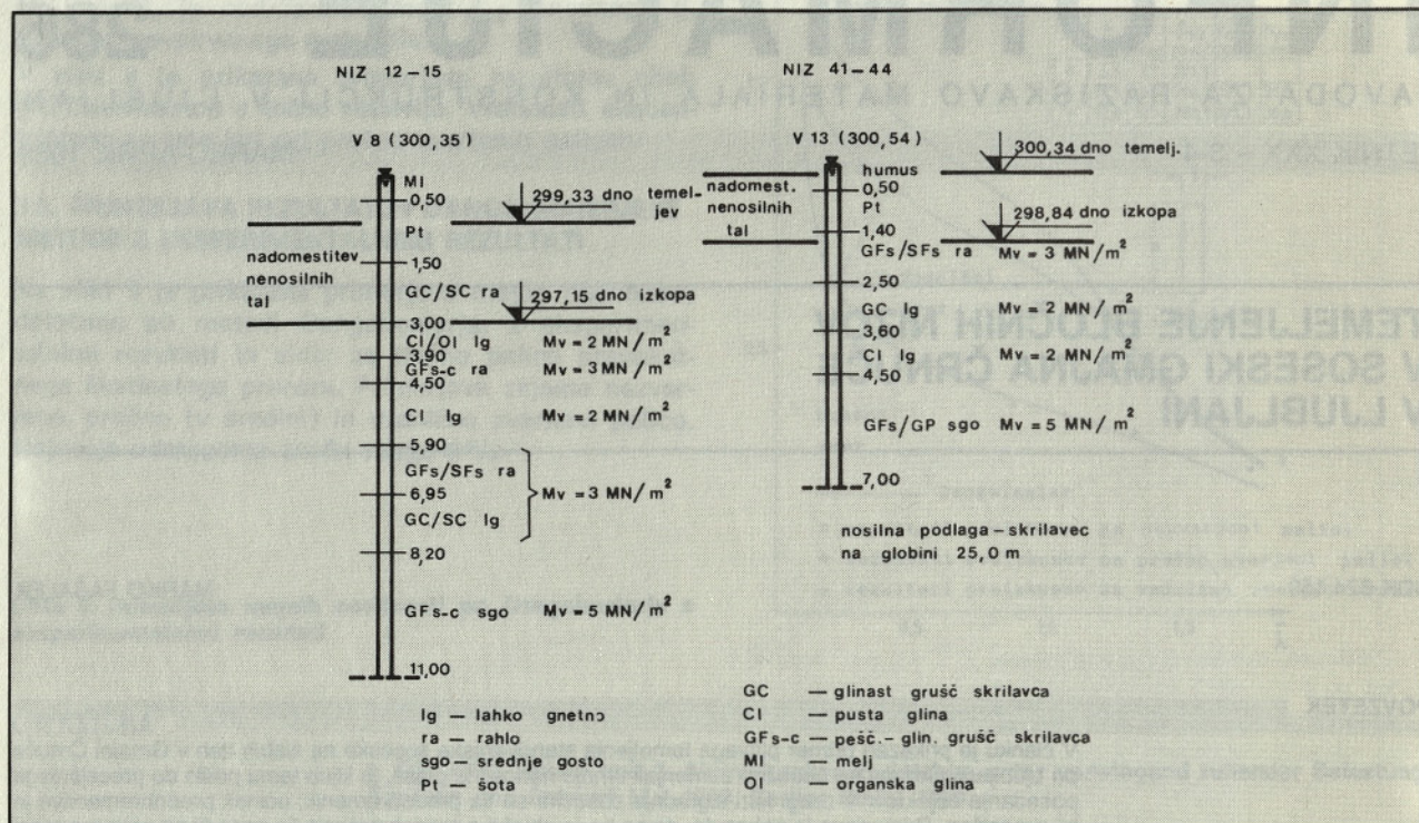
Slika 1. Sestava tal
