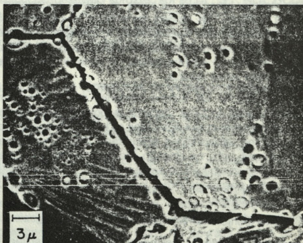
Slika 2. Interkristalno napetostno pokanje zaradi številnih depozitov po kristalnih mejah zrn
