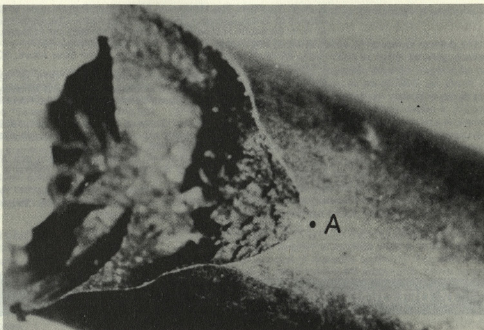
Slika 10: Prelomna površina napetostne korozijske razpoke patentirane žice
