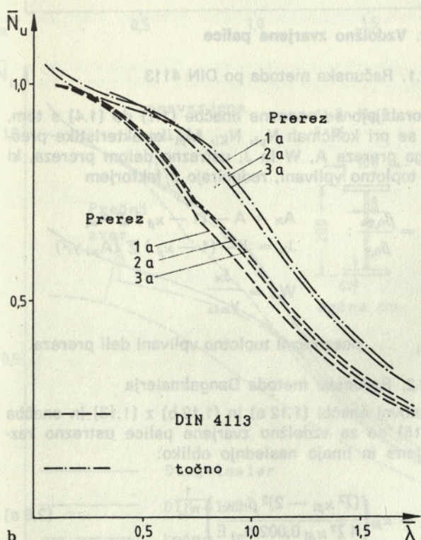
Slika 5. Primerjava mejne nosilnosti nezvarjenih tlačnih palic, določene po Dangelmaierjevi metodi in DIN 4113 s točnimi vrednostmi
