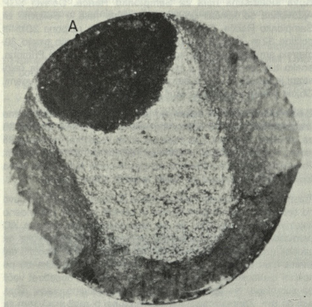
Slika 11. Videz prelomne površine poboljšane Dywidag jekla, ki je počilo zaradi delovanja napetostne korozije
