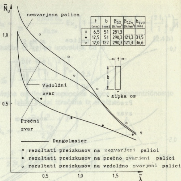
Slika 9. Primerjava mejnih nosilnosti po Dangelmaierju z eksperimentalnimi rezultati
